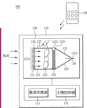
微型清淨機模組
